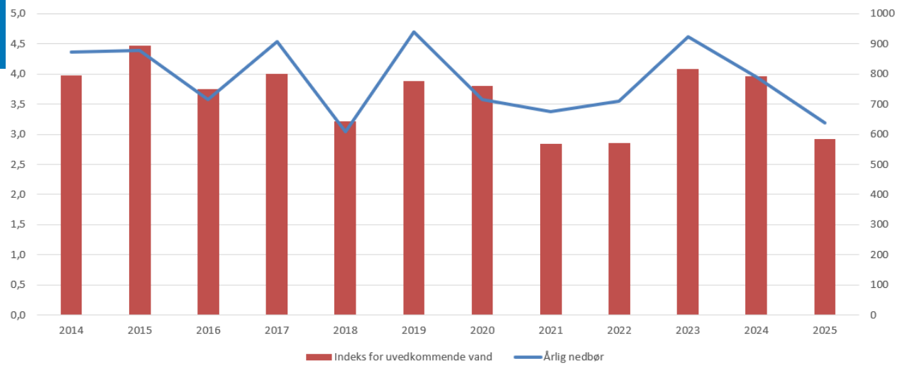
Spildevand - oversigt over vandmængder
